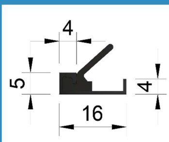
Maatvoering
